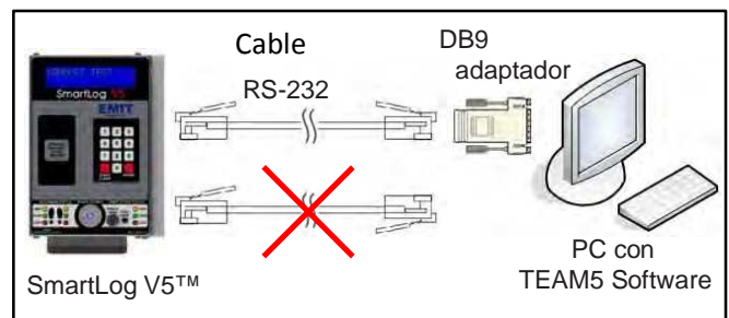
Figura 21. Conexión directa del SmartLog V5™ a un PC
