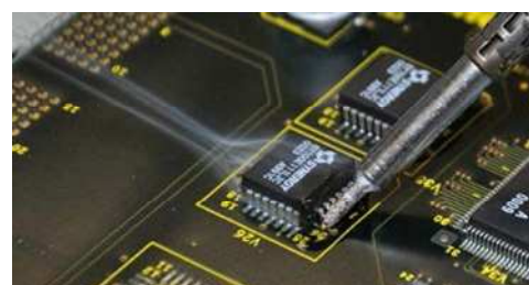
Extracción de humos directa desde la unión de soldadura
